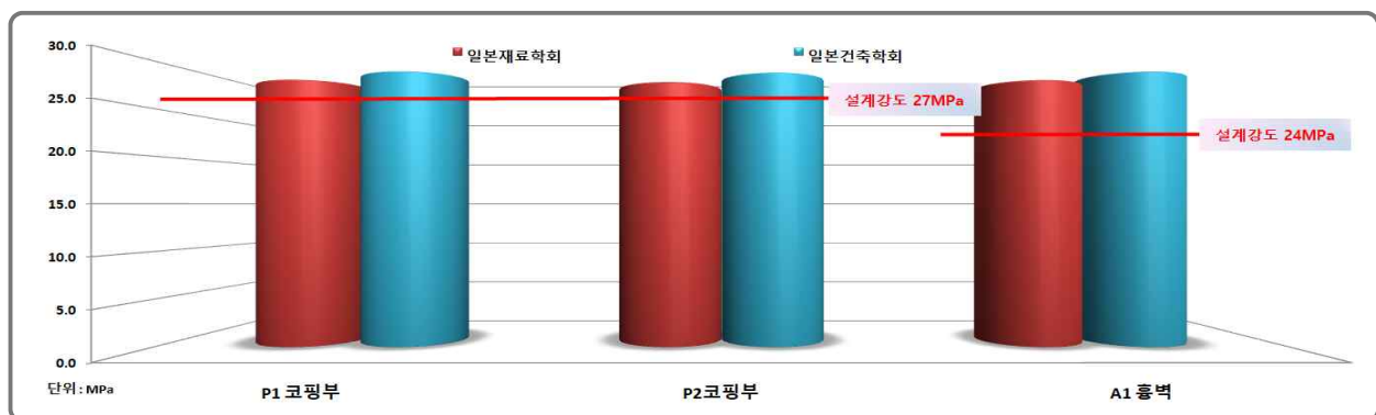
[그림 4.2.3] 반발경도법에 의한 비파괴강도 측정 결과-하부구조
