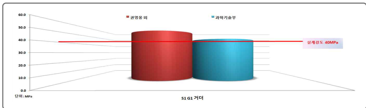
[그림 4.2.2] 반발경도법에 의한 비파괴강도 측정 결과-상부구조(거더)
